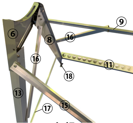
A矢視
