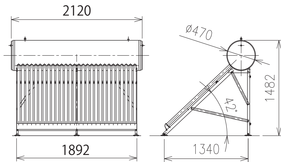
標準寸法図
