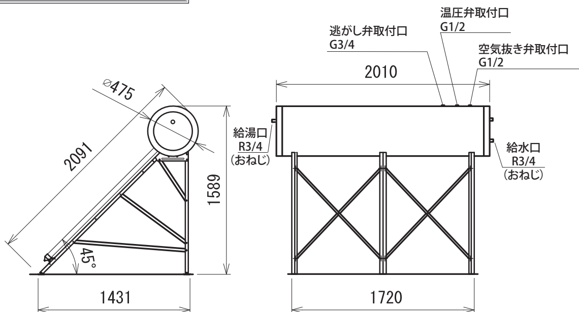
標準寸法図 ST-195/24F-Y
